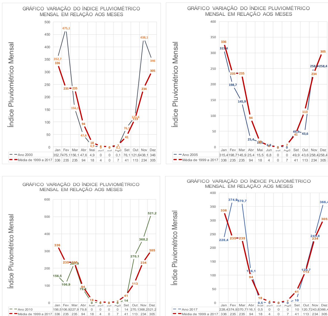
Figura 2: Índice Pluviométrico, Estação Nova América, 2000, 2005, 2010 e 2017.
